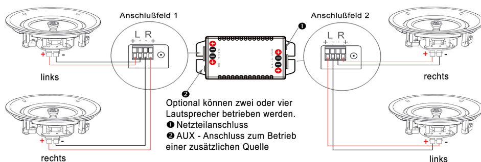
Anschlussschema für zalias AMP4X15BT Lautsprecher am 4-Kanal Bluetooth®
